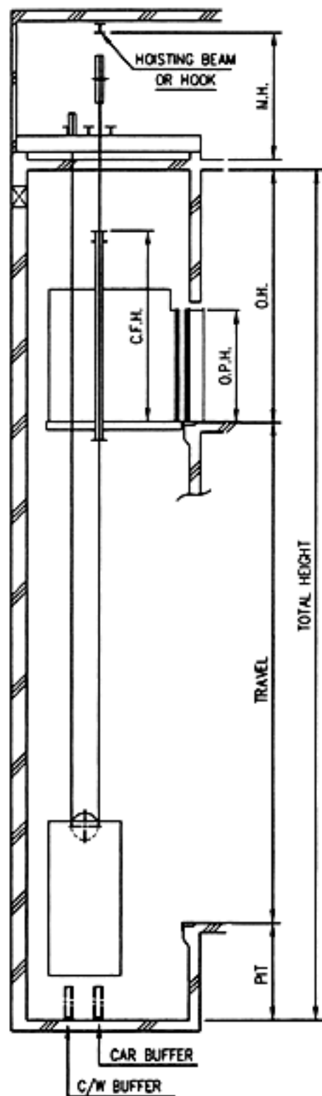
HOISTWAY ELEVATION
