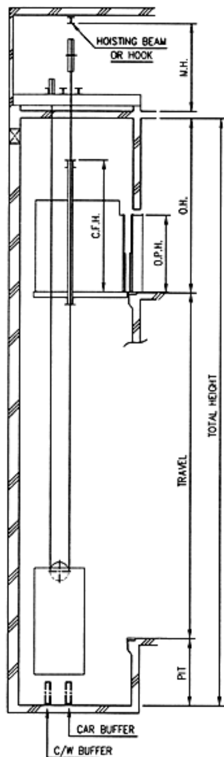
HOISTWAY ELEVATION
